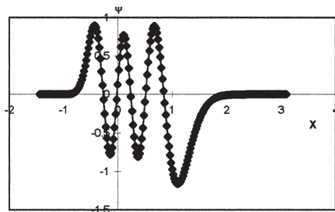
图 13.2: 通过 Numerov 方法求出的 \text{H}_2 v = 5 莫尔斯振动波函数。
